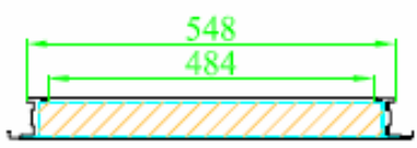
Sección B-B
